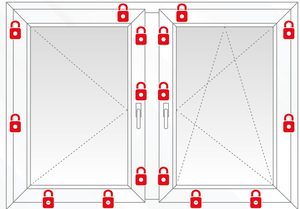
Die Anzahl der Pilzzapfen hängt vom Aufbau und den Massen des Fensters ab.
